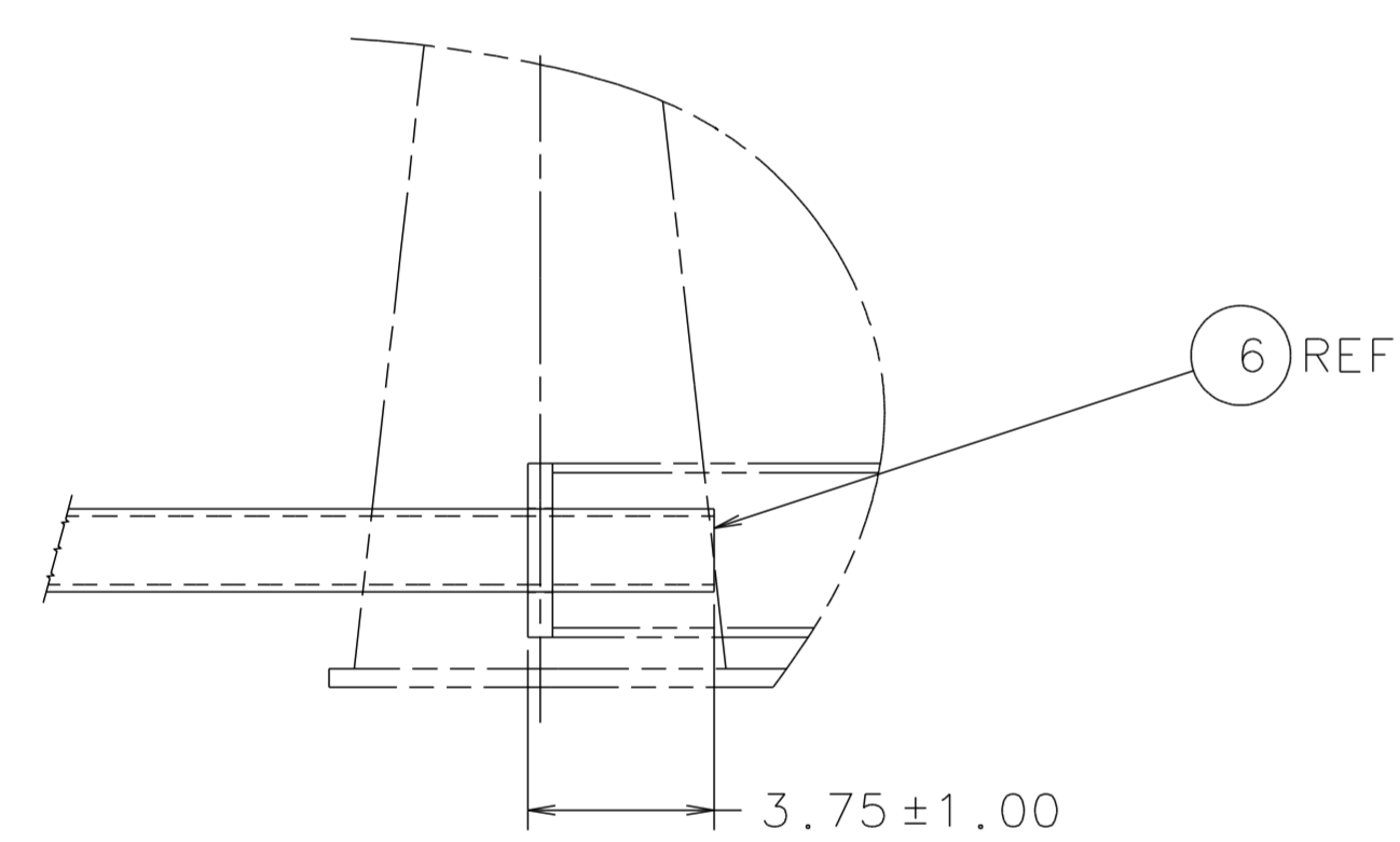
VIEW C SCALE: 1/4
