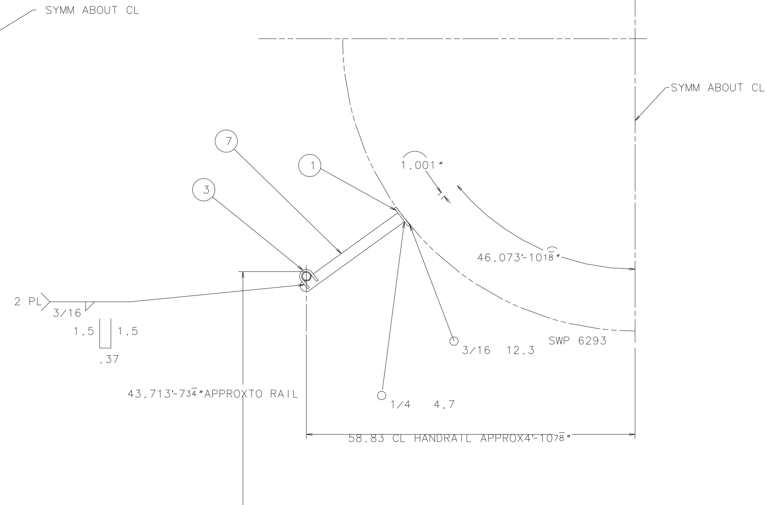
SECTION D-D SCALE: 1/8 2 PL
